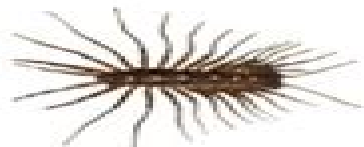
Scutigeroforms
