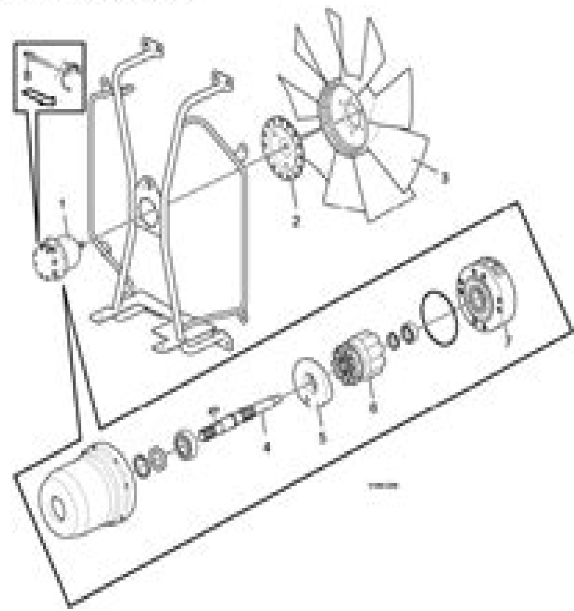
Figure 1 Cooling fan motor and fan
