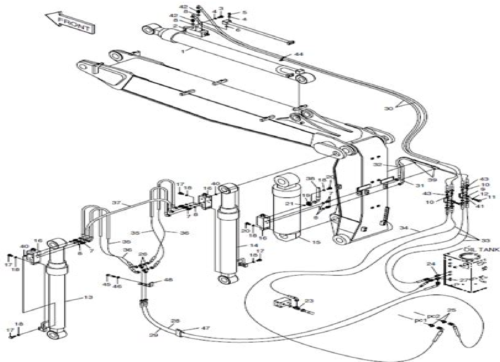
Fig. 6990 LOCK VALVE PIPING-ARTILBOOM CONDUITES DE VERROU VANNE
