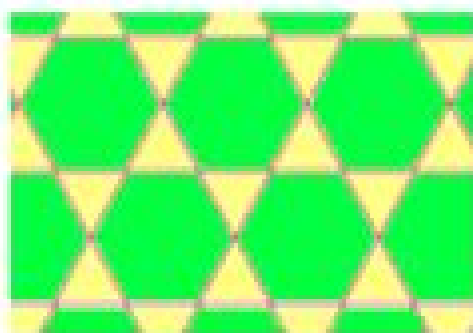
3.6.3.6
