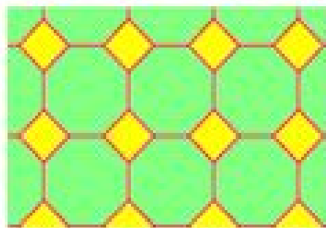
4.8.8
