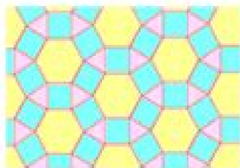
3.4.6.4
