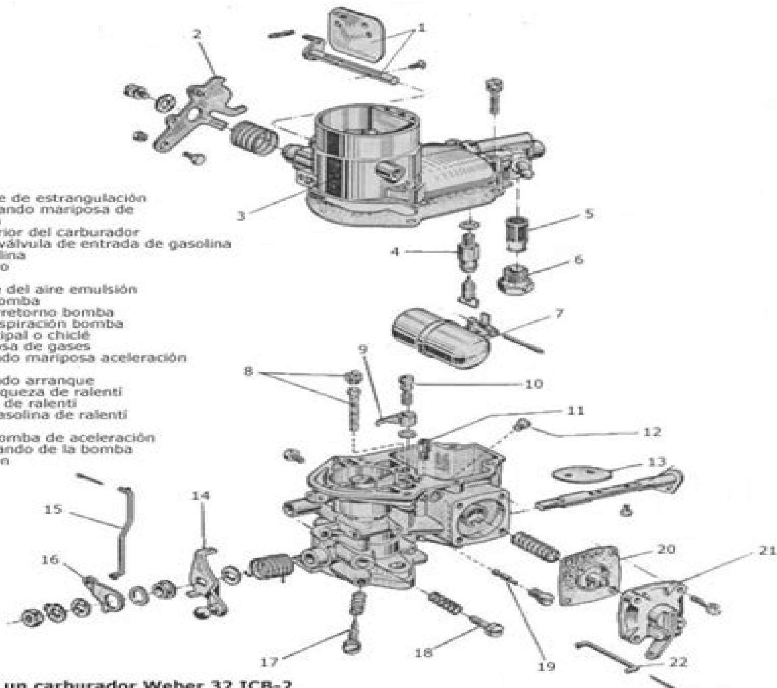
Despiece de un carburador Weber 32 ICB-2
